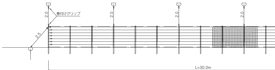
簡易アングルフェンス工設置図(土中用タイプ)
